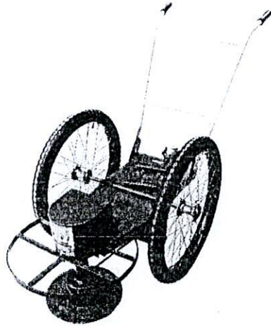
รถเข็นค้ำหน้าสามล้อใหญ่ 2 ล้อ เกลือกอม (โครง), 2 ล้อ เกลือกเลื่อน (โครง)
