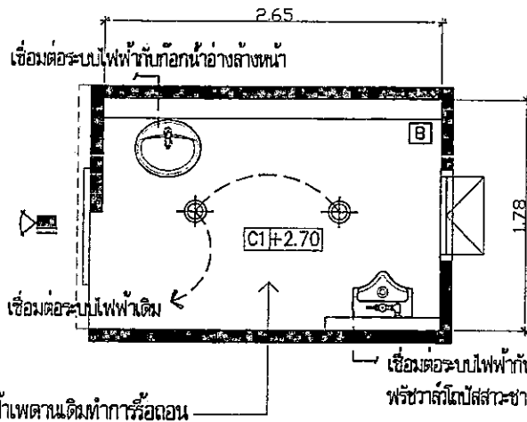
แปลนระบบไฟฟ้า
