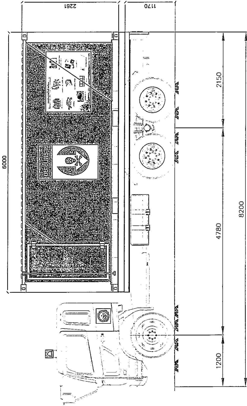
รูปแบบตัวอย่างด้านข้าง(ซ้าย)รถบรรทุกขยะอันตราย
