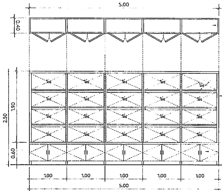
รูปด้านตึกข้างของ
