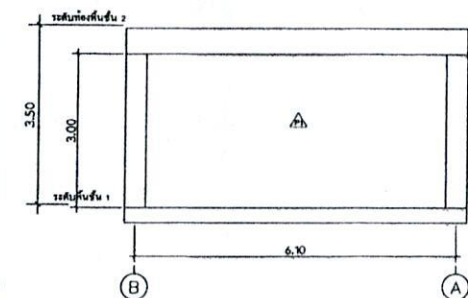
แบบรูปตาดัน 4 ขนาดพิมพ์ 1 : 75
