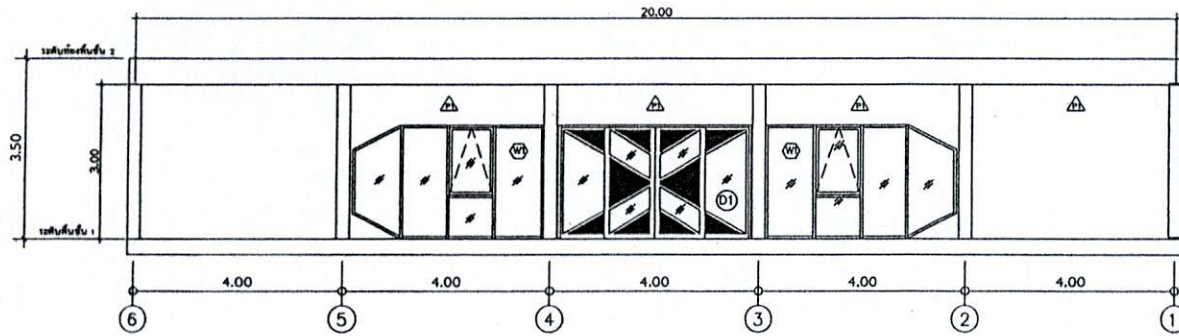
แบบรูปตาดัน 1 ขนาดพิมพ์ 1 : 75
