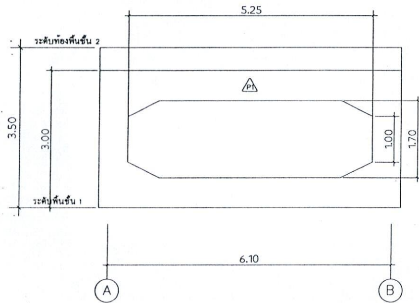
แบบขยายผนัง ตกแต่งแปดเหลี่ยม
