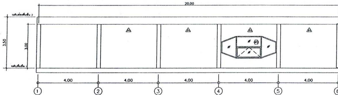
แบบรูปตาดัน 3 ขนาดพิมพ์ 1 : 75
