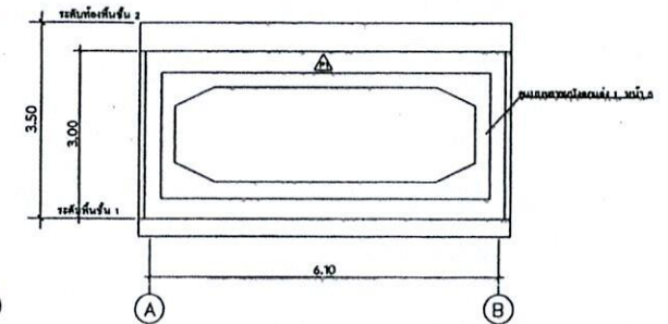
แบบรูปตาดัน 2 ขนาดพิมพ์ 1 : 75
