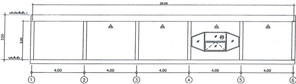
แบบรูปด้าน 3 มาตราส่วน 1 : 75
