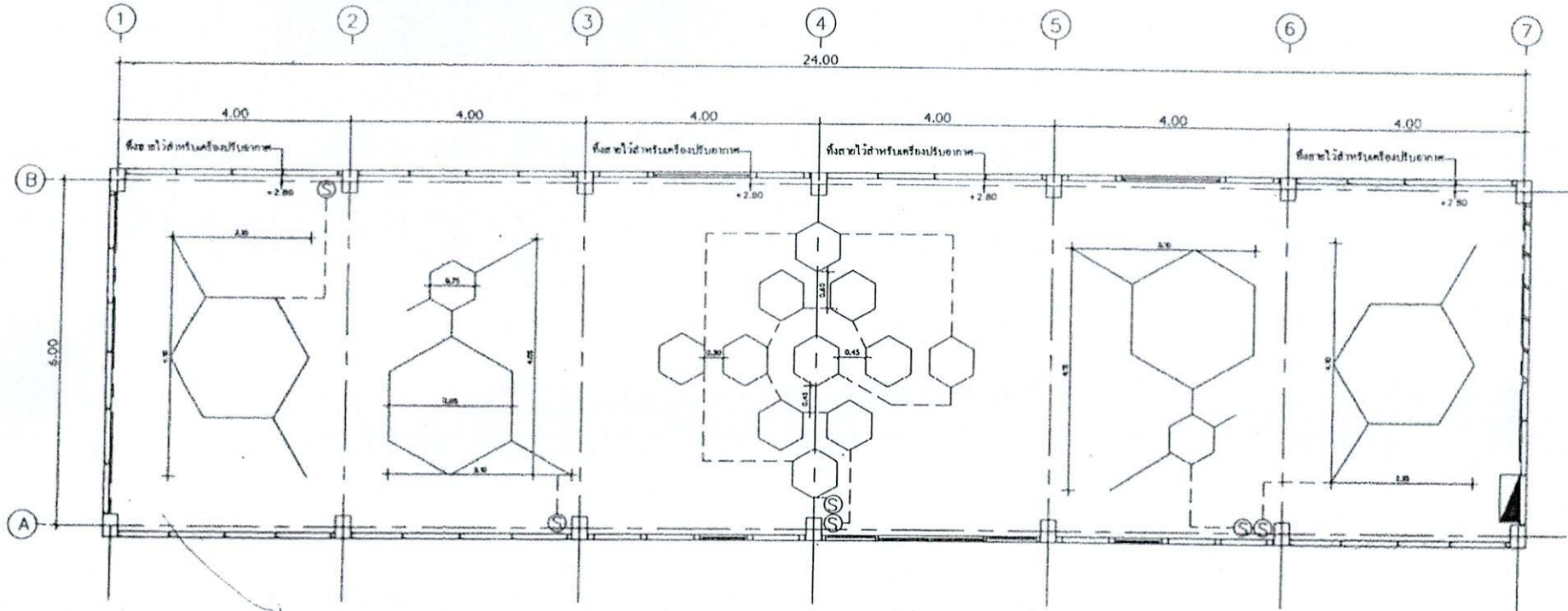
รายการประกอบแบบไฟฟ้า
