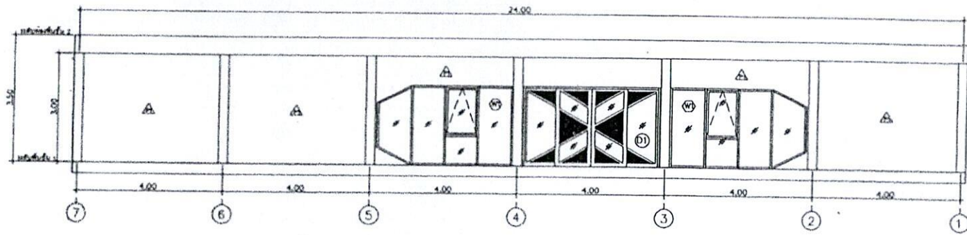
แบบรูปตึก 1 มาตราส่วน 1 : 75
